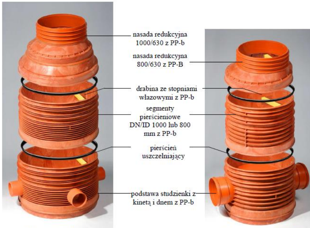
Rys.2 Studzienka PRO 1000
